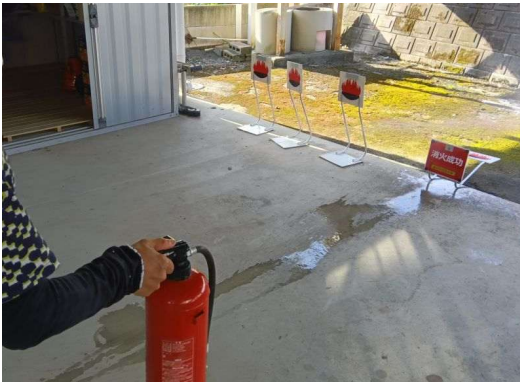
7 * 水消火器による訓練
